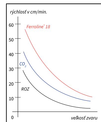
Pomer rýchlostí zvarovania v ochrannej atmosfére CO 2 , FERROLINE® C18 a ROZ.
