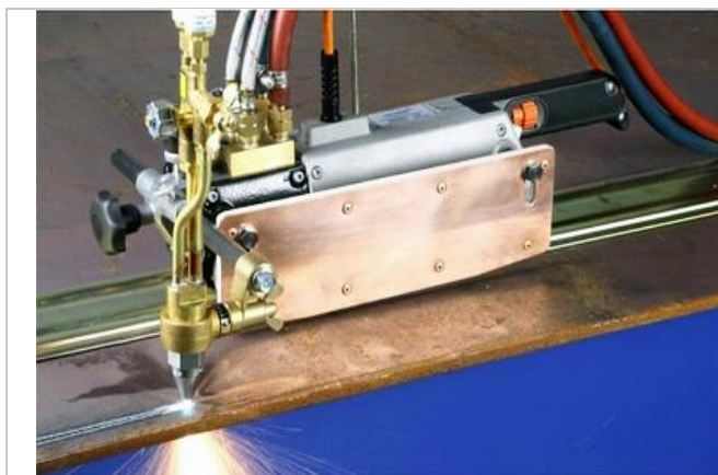
S jedným strojným rezacím horákom
