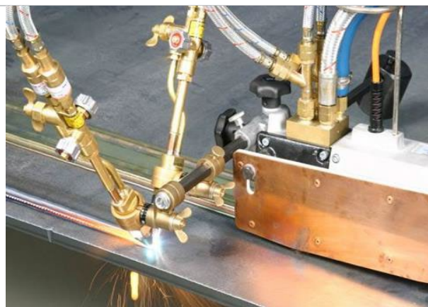
S dvoma strojnými rezacími horákmi
